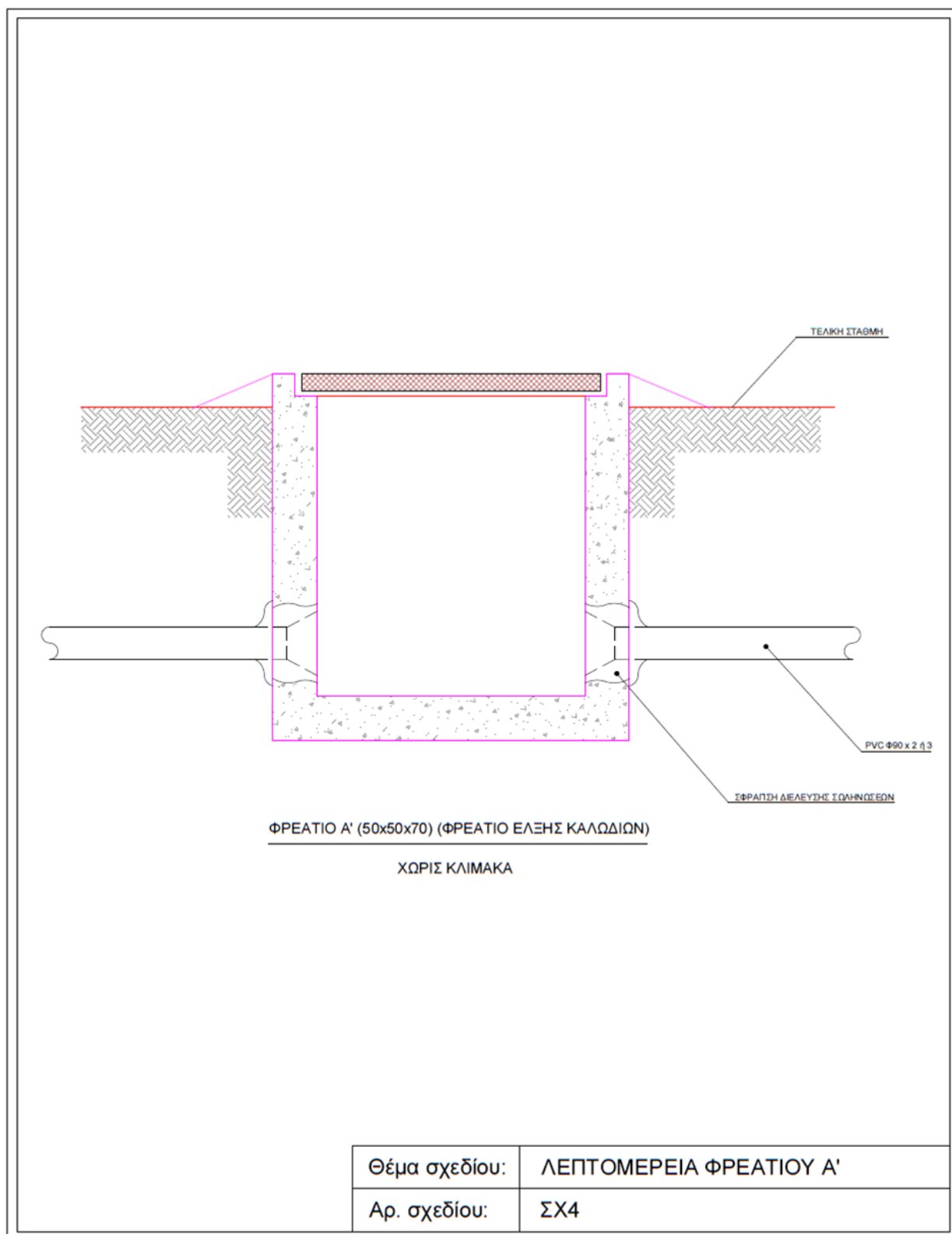
Εικόνα 4. Σχέδιο Λεπτομέρειας Φρεατίου Α'
