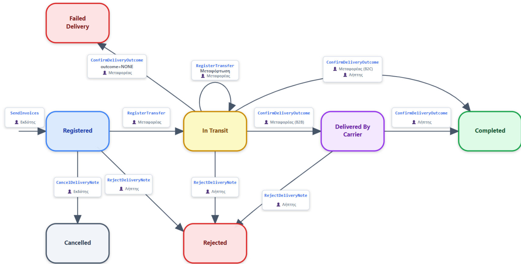
Εικόνα 1: Διάγραμμα Καταστάσεων
