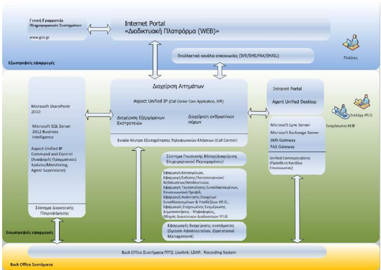
Δομικά Στοιχεία - Αρχιτεκτονική «Κέντρου Εξυπηρέτησης Φορολογουμένων»
